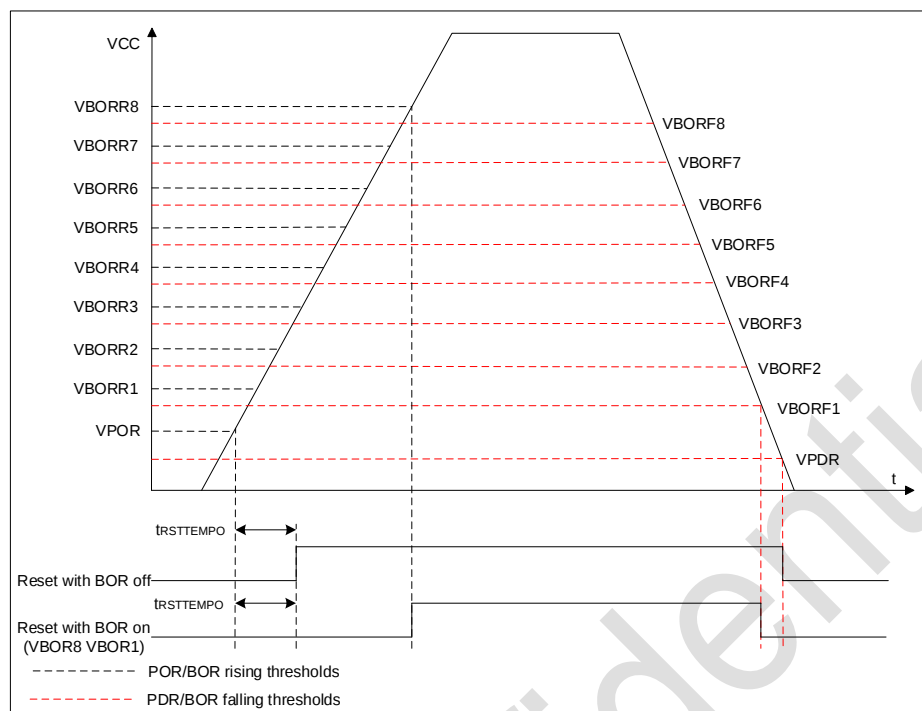
图 2-3 POR/PDR/BOR 阈值
