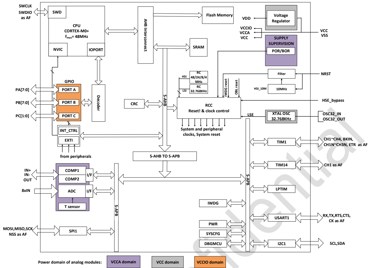
图 1-1 功能模块
