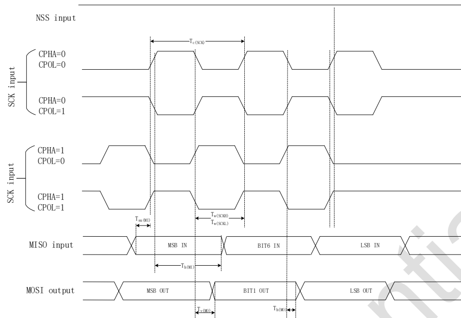
图 5-6 SPI 时序图-master mode
