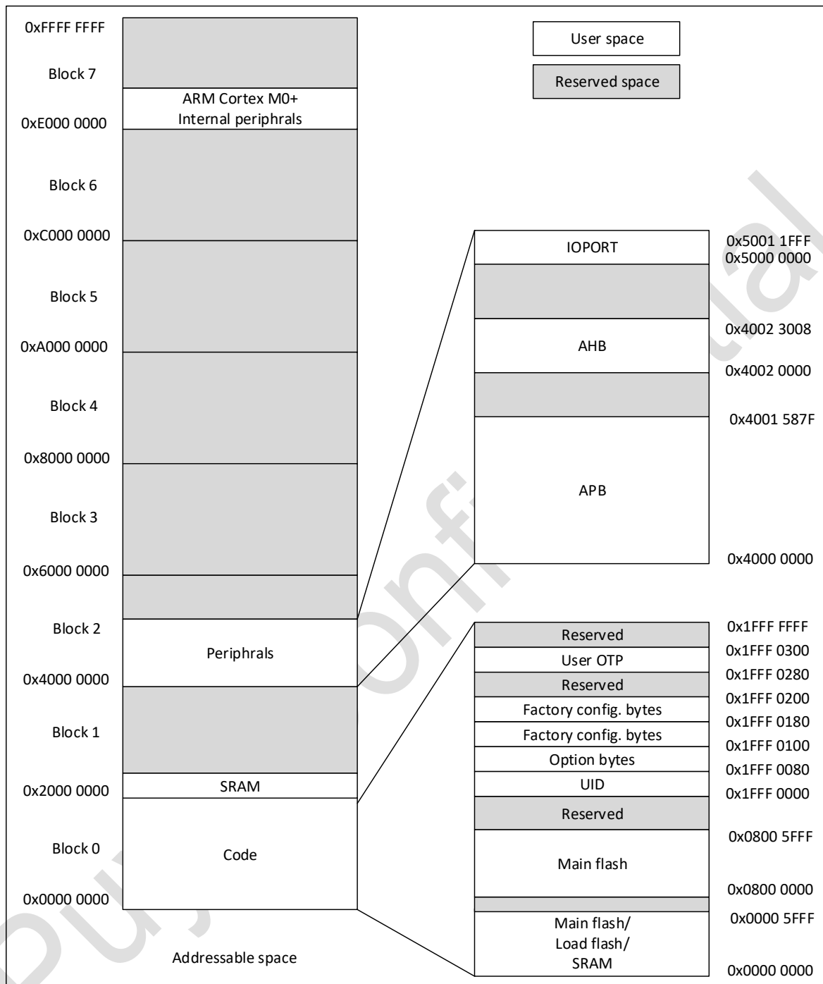
图 4-1 存储器映射
